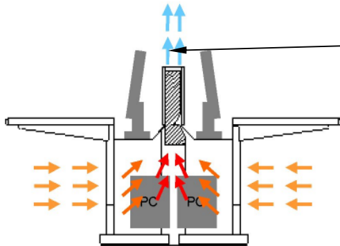
Handelaarstafel met smalle TFT beeldschermen, slechts weinig plaats voor fancoil aanwezig.
